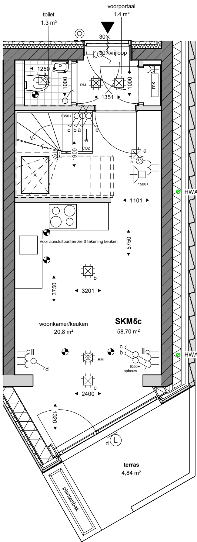
begane grond
