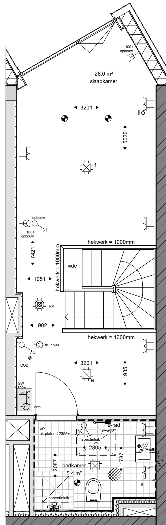
eerste verdieping
