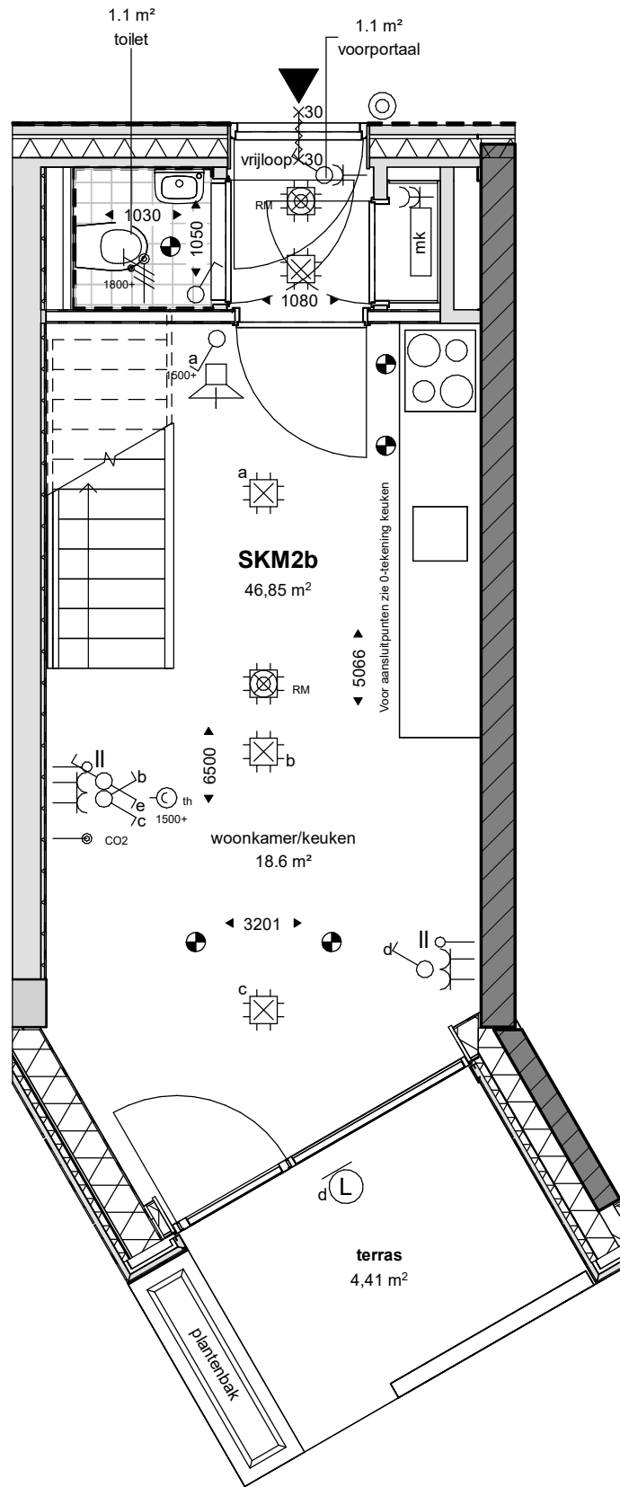
begane grond
