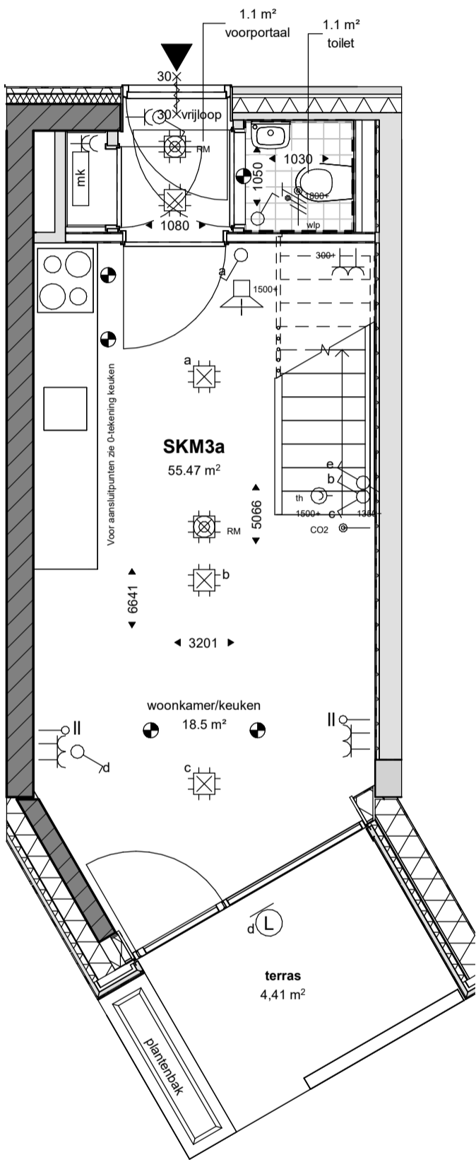
begane grond
